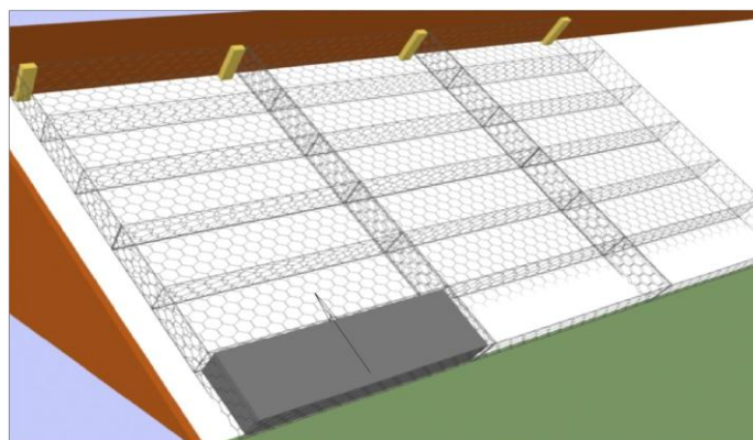
Рисунок 5.4.7 – Установка и заполнение ГСИ на склоне
