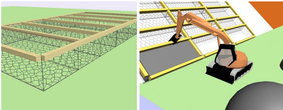
Рисунок 5.4.8 — Вид ГСИ подготовленного для механизированного заполнения
