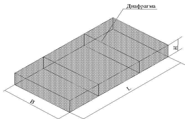
Рисунок.1. Размеры ГСИ.
